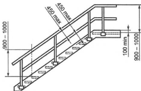
Рисунок 4. Геометрические параметры Расположение поручней на защитного ограждения маршевой лестницы. угол наклона от 55^{\circ} до 75^{\circ} .
