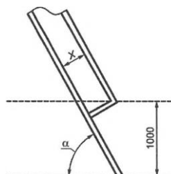
Рисунок 4. Геометрические параметры Расположение поручней на защитного ограждения маршевой лестницы. угол наклона от 55^{\circ} до 75^{\circ} .
