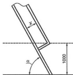
Рисунок 4. Геометрические параметры Расположение поручней на защитного ограждения маршевой лестницы. угол наклона от 55^{\circ} до 75^{\circ} .
