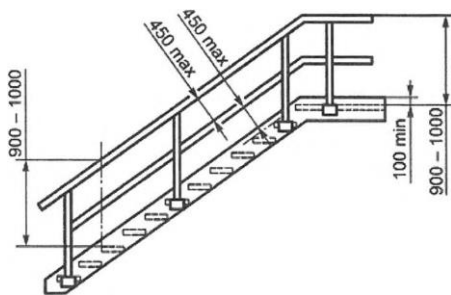
Рисунок 4. Геометрические параметры Расположение поручней на защитного ограждения маршевой лестницы. угол наклона от 55^{\circ} до 75^{\circ} .
