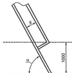
Рисунок 4. Геометрические параметры поручней на защитного ограждения маршевой лестницы. 75^\circ .
