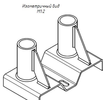
Изометричный вид М1:2
